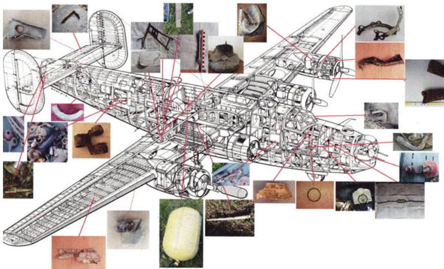
A megtalált alkatrészek eredeti helye a gépen
